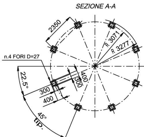
MODELLO CAMS 8CS6 CAPACITA' 320mc
