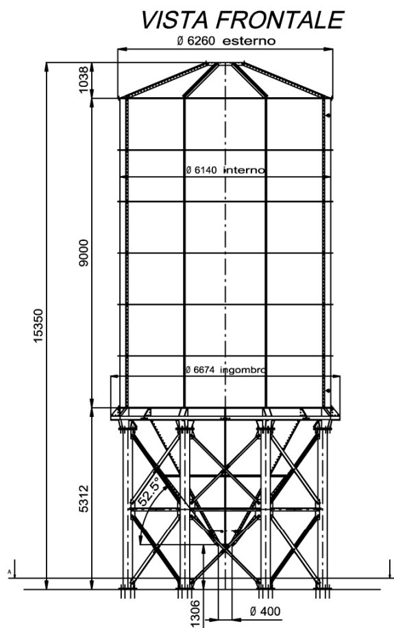
MODELLO CAMS 8CS6 CAPACITA' 320mc
