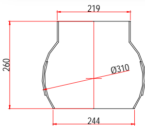
Codice. 28.050.1219 Bocca sferica regolabile coclea Ø 219 per calza gomma para
