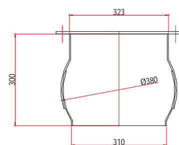
Codice 28.050.1824 Bocca sferica flangiata per coclea Ø 323 c/flangia Cod. 27.001.1410
