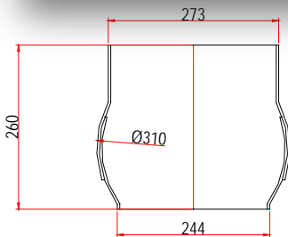
Codice 28.050.1273 Bocca sferica regolabile coclea Ø 273 per calza gomma para
