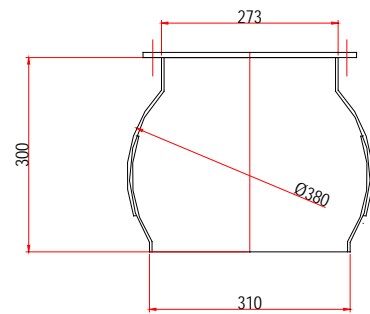
Codice 28.050.1776 Bocca sferica flangiata per coclea Ø 273 c/flangia Cod. 27.001.1330
