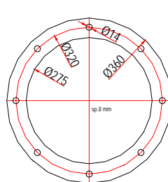
Codice 28.050.1719 Bocca sferica flangiata per coclea Ø 219 c/flangia Cod. 27.001.1282
