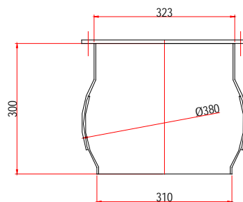
Codice 28.050.1823 Bocca sferica flangiata per coclea Ø 323 c/flangia Cod. 27.001.1380
