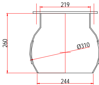
Codice 28.050.1719 Bocca sferica flangiata per coclea Ø 219 c/flangia Cod. 27.001.1282
