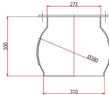
Codice 28.050.1775 Bocca sferica flangiata per coclea Ø 273 c/flangia Cod. 27.001.1360
