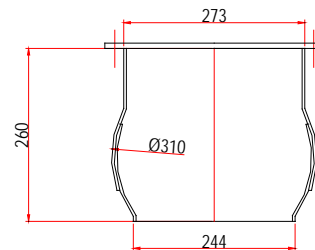
Codice 28.050.1774 Bocca sferica flangiata per coclea Ø 273 c/flangia Cod. 27.001.1360
