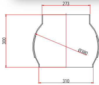
Codice 28.050.1274 Bocca sferica regolabile coclea Ø 273 per calza gomma para
