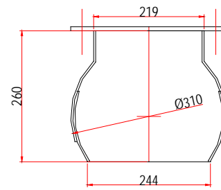
Codice 28.050.1720 Bocca sferica flangiata per coclea Ø 219 c/flangia Cod. 27.001.1310
