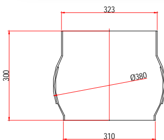
Codice 28.050.1323 Bocca sferica regolabile coclea Ø 323 per calza gomma para
