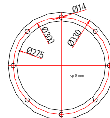
Codice 28.050.1720 Bocca sferica flangiata per coclea Ø 219 c/flangia Cod. 27.001.1310
