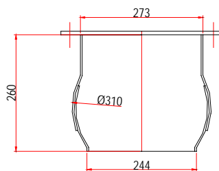
Codice 28.050.1773 Bocca sferica flangiata per coclea Ø 273 c/flangia Cod. 27.001.1330
